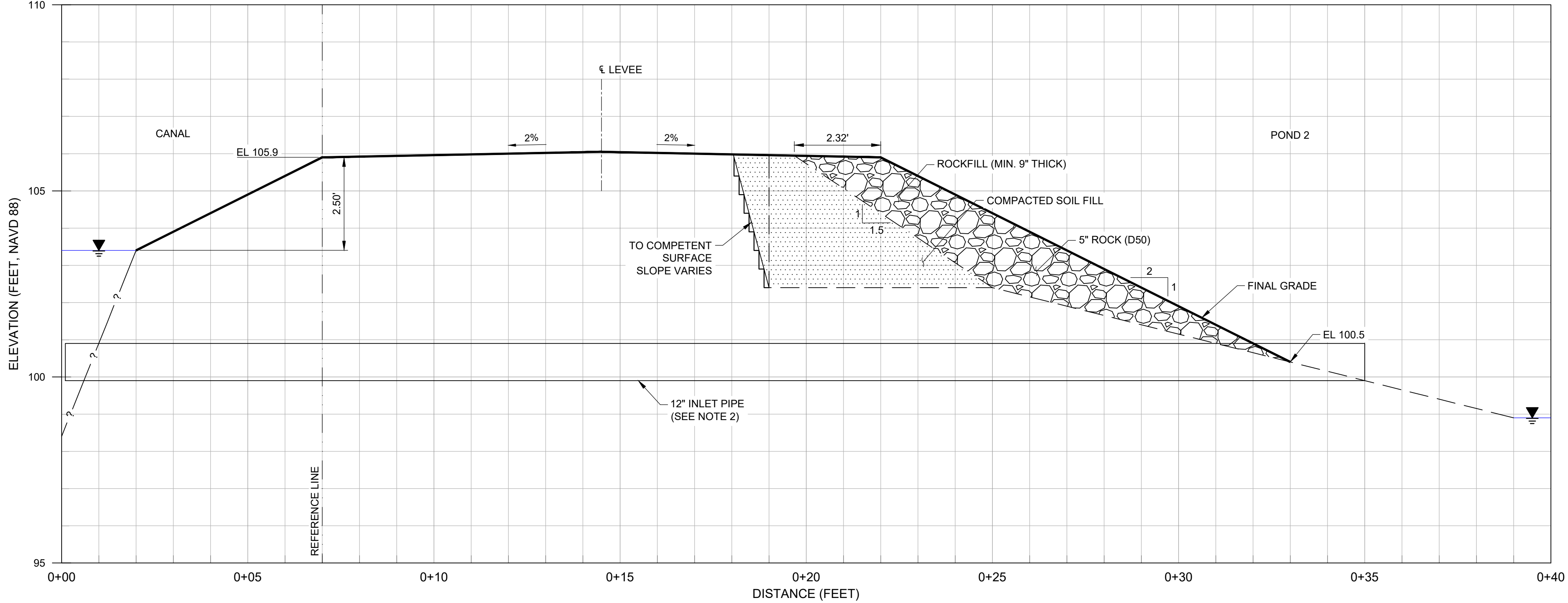
TYPICAL SECTION - REACH 5 - STA 245+00 TO STA 935+00 SCALE: 1" = 2'
