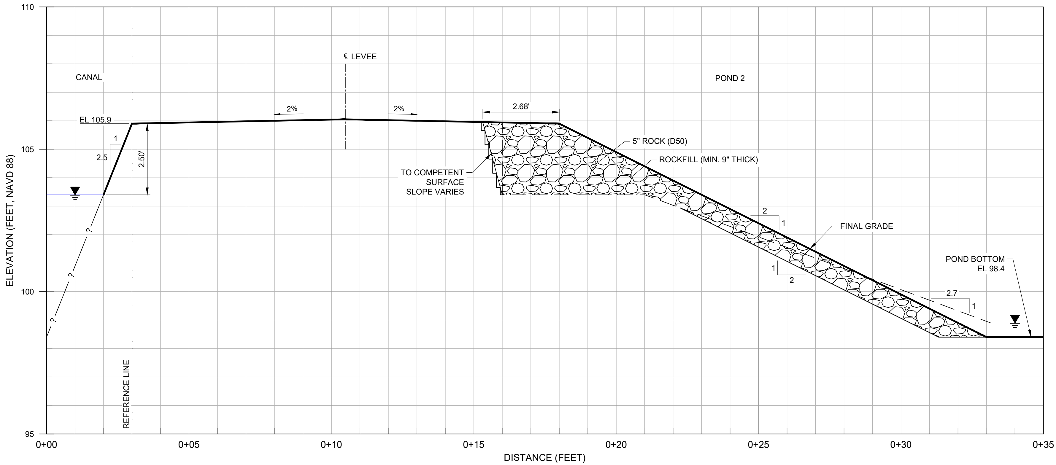
TYPICAL SECTION - REACH 4 - STA 230+00 TO STA 245+00 SCALE: 1" = 2'
