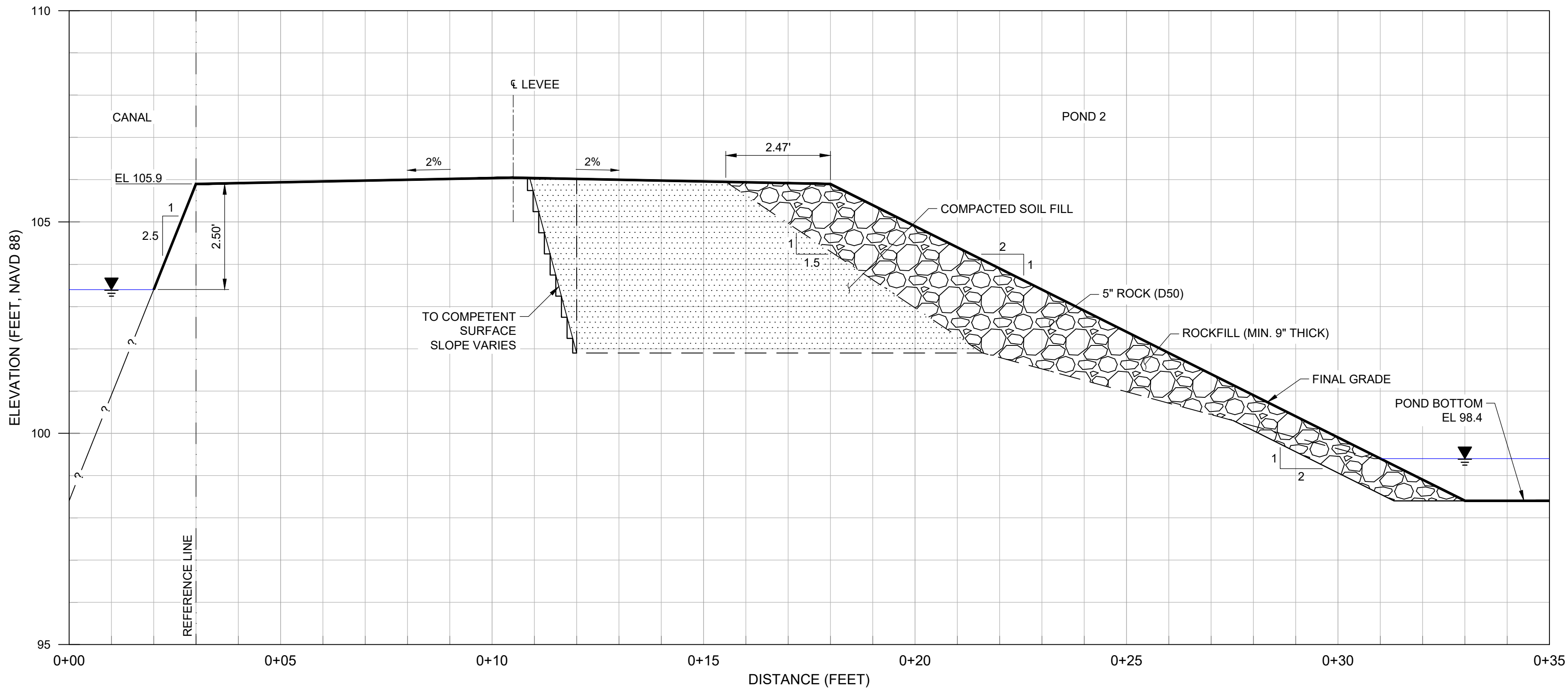
TYPICAL SECTION - REACH 3 - STA 219+40 TO STA 230+00 SCALE: 1" = 2'
