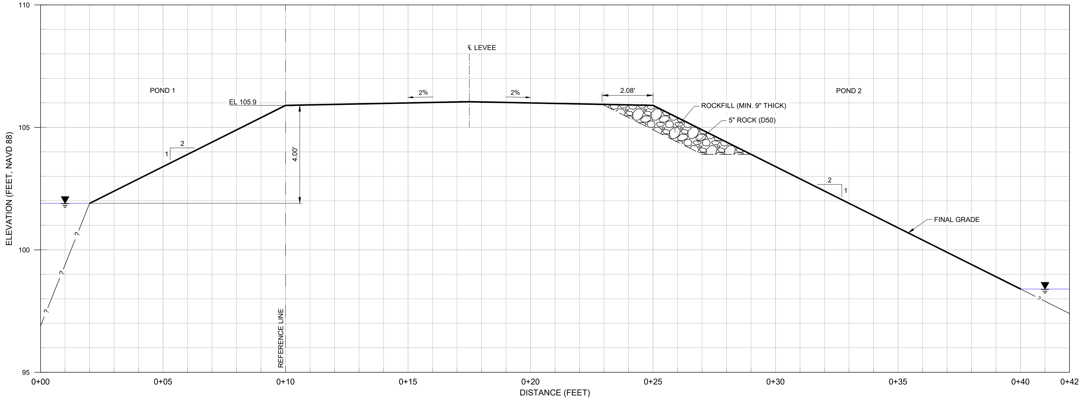
TYPICAL SECTION - REACH 6 - STA 935+00 TO STA 912+00 SCALE: 1" = 2'
